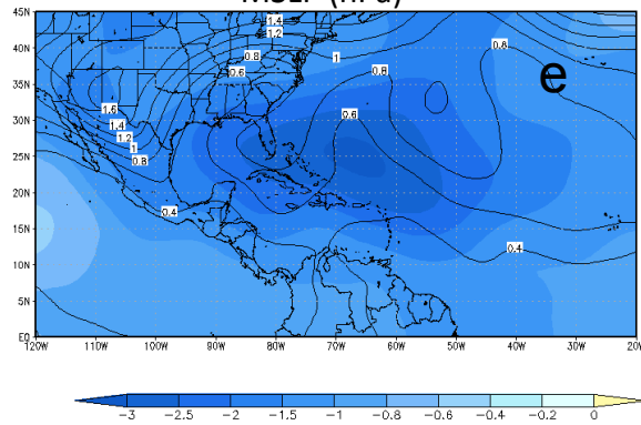
MSLP (hPa)
