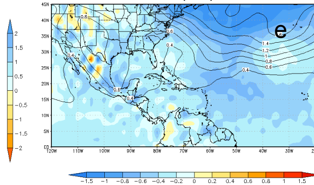
MSLP (hPa)
